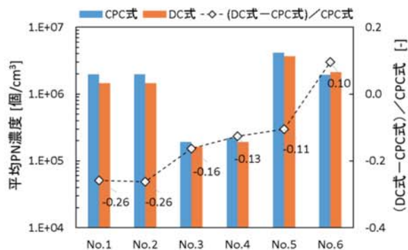
図3 各 PN PEMS による平均 PN 濃度
