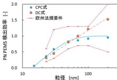
図4 各 PN PEMS の検出効率
